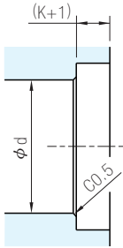
DWD段付形座金 加工尺寸
